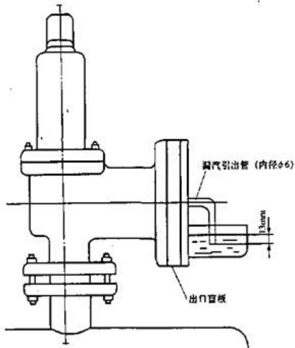
图 1 常温密封性能装置图
