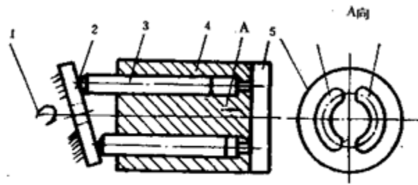
1—传动轴；2—斜盘；3—柱塞；4—缸体；5—配油盘
