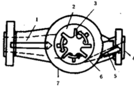
1—吸入口； 2—环形空间； 3—叶轮； 4—压出口； 5—扩散锥管； 6—喷嘴； 7—泵体
